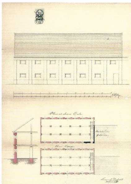
14. KÉP: Kőbánya, Baumann Károly maglárterv (BFL XV 17/b.312. Pest város Építő Bizottmánya 62/1862.) Budapest Főváros Levéltára engedélyével
