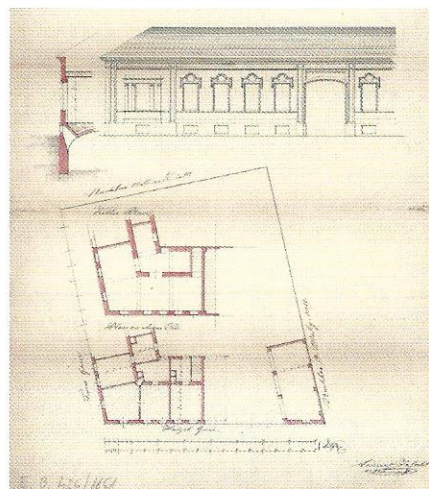
15. KÉP: Ferencváros, Berzenczey utca. Frankovics Ferenc ház tervrajz (BFL XV 17/b.312. Pest város Építő Bizottmánya 425/1861). Budapest Főváros Levéltára engedélyével
